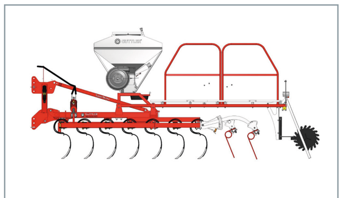
Option: Sägerät pneumatisch für Zwischenfrüchte. Zweite Reihe Striegel.
