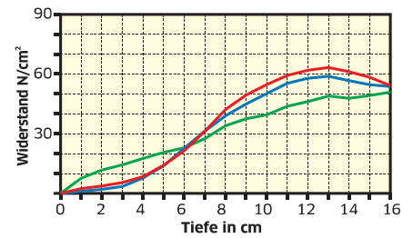
Rückverdichtungskurven der Simplex Prismenwalze®
